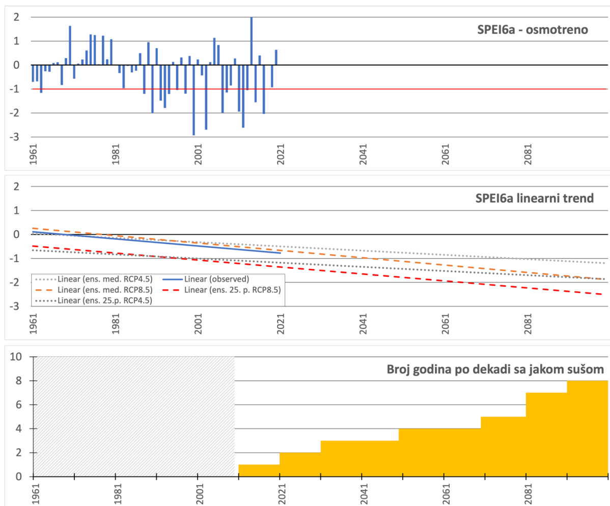
Слика Д1.11. Вредност SPEI6a за сваку годину у периоду 1961-2020 (горњи панел), линерани тренд SPEI6a за период 1961-2011 из осматрених вредности, и пројектоване вредности ансамблом модела (средњи панел) по RCP4.5 и RCP8.5 сценаријима (медијане и вредности 25. перцентила ансамбла модела), и учесталост година са јаким сушама по декади у периоду 2011-2100 добијених из пројекција ансамбла модела по RCP8.5 сценарију (доњи панел).
