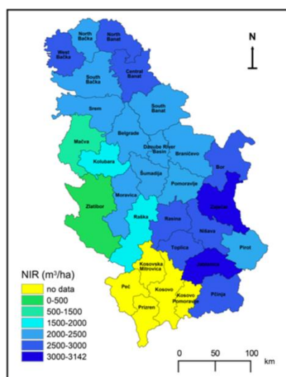
Слика Д2.33. Процењена вредност нето нормe наводњавања по областима у Србији, узимајући метеоролошке параметре у по једној репрезентативној локацији за сваки округ. Процењене вредности су просек за климатски период блиске прошлости, односно за 2000-2019 (до када су били на располагању подаци у време када је рађена процена).
