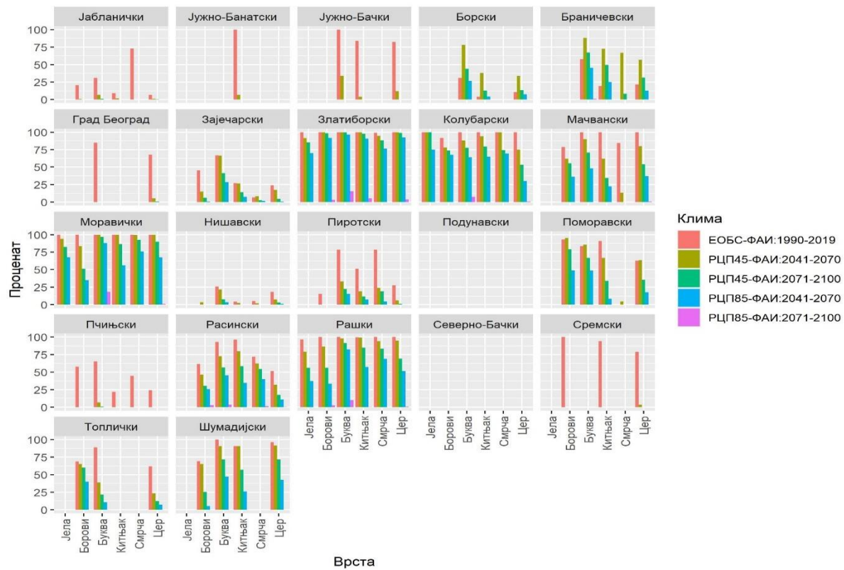
Слика Д3.2. Проценат погодних станишта за јелу, борове, букву, китњак, смрчу и цер по административним областима у Републици Србији. Процене добије по FAI индексу.
