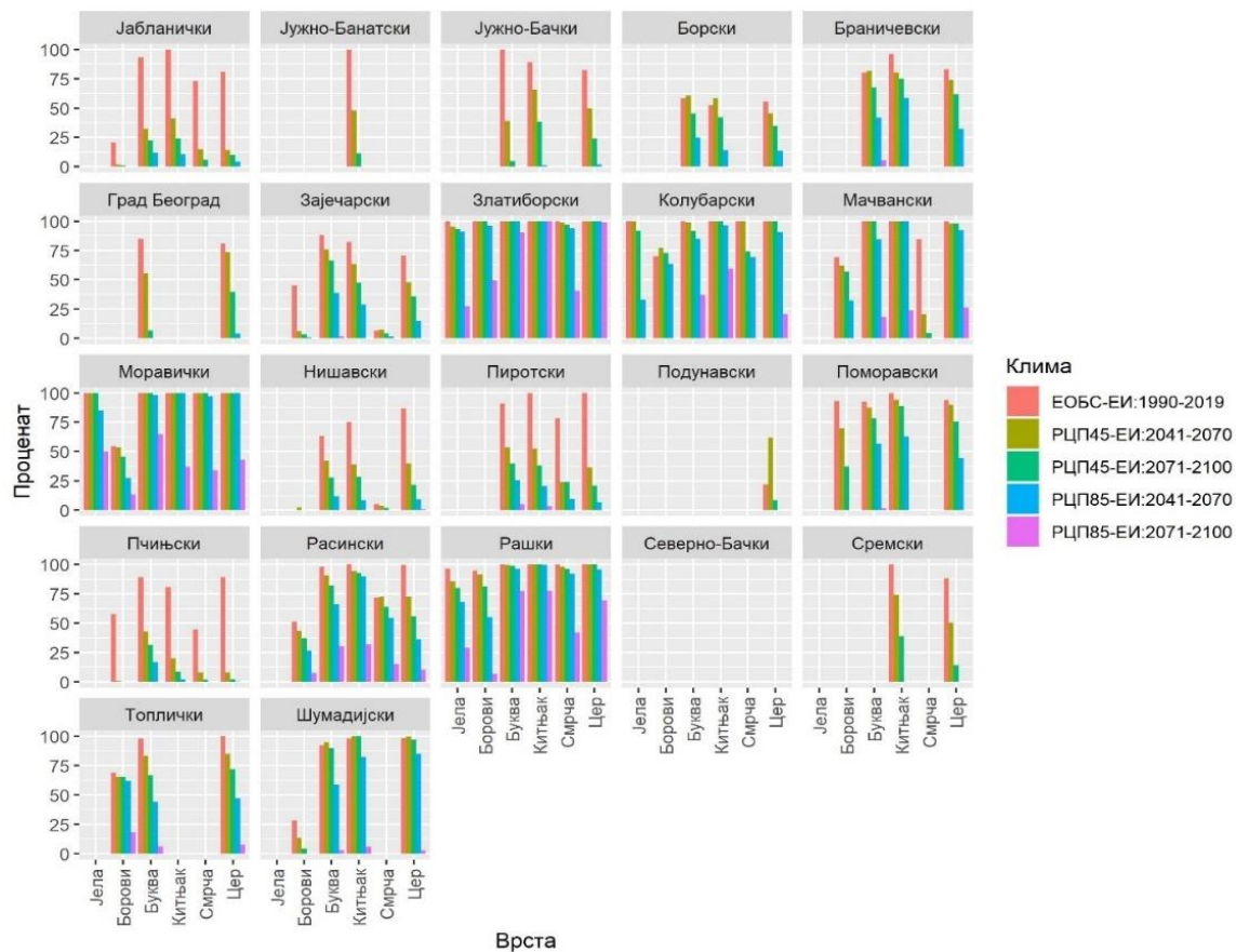
Слика ДЗ.1. Процент погодних станишта за јелу, борове, букву, китњак, смрчу и цер по административним областима у Републици Србији. Процене добијене по Еленберговом индексу
