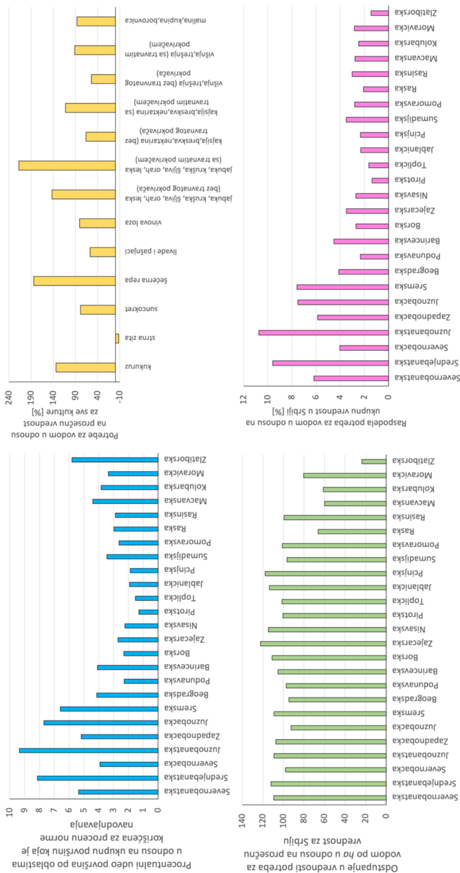
Слика Д2.34. Процентуални удео површина по областима које су узете у процени нето нормe наводњавања у односу на укупну површину узету у обзир у овој процени у Републици Србији (панел горе лево). Просечне потребе за водом на територији Републике Србије за одређене групе култура и за ливаде и пањњаке (панел горе десно). Процентуални удео потреба за водом по областима по хектару у односу на просечне потребе по хектару разматраних култура гајених на територији Републике Србије (панел доле лево). Процентуални удео потреба за водом по областима у односу на укупну потребу на територији Републике Србије (панел доле десно). Ове процене су израђене за климатски период 2000–2019, где су једини временски променљиви подаци метеоролошке величине.
