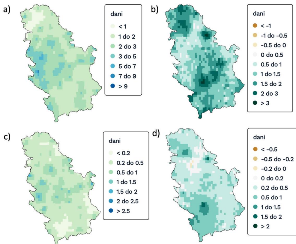
Слика Д1.8. Средњи број дана по години са веома јаким и екстремно јаким падавинама - дани са падавинама преко 20mm за 1961-1990 (горе лево) и промена броја ових дана за 2001-2020 у односу на 1961-1990 (горе десно), и средњи број дана са екстремно јаким падавинама – дани са падавинама преко 30mm за 1961-1990 (доле лево) и промена броја ових дана за 2001-2020 у односу на 1961-1990 (доле десно).
