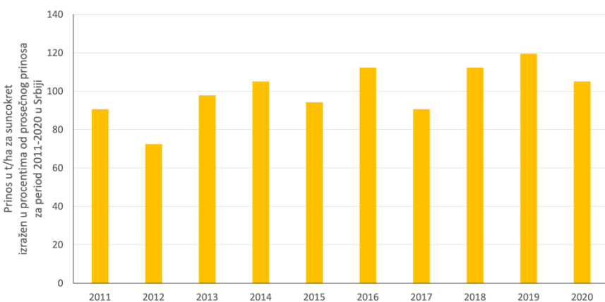
Слика Д2.18. Проценат од просечног приноса сунцокрета у t/ha у периоду 2011-2020 за сваку годину на територији Републике Србије.
