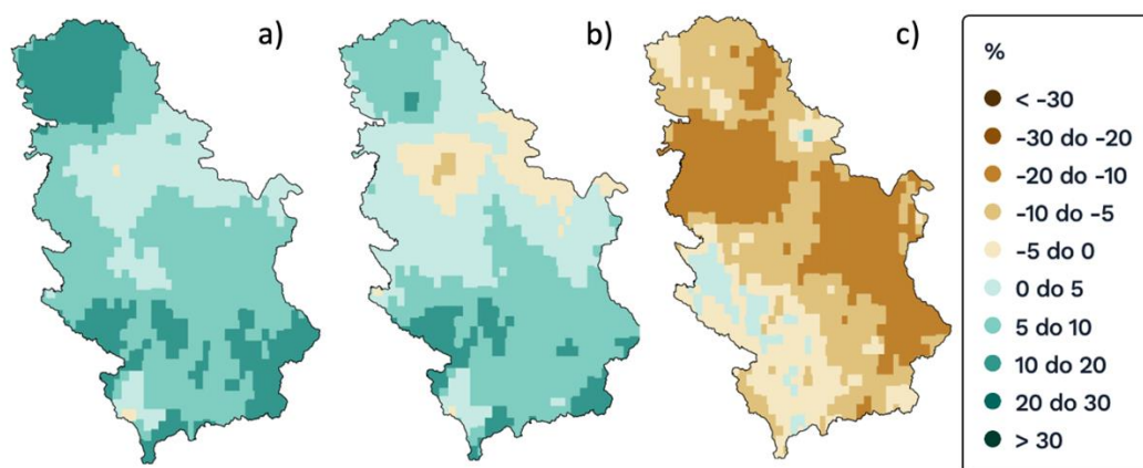
Слика Д1.6. Промена годишњих сума падавина за 2001-2020 (лево) и 2011-2020 (средње) у односу на 1961-1990, и сума падавина за ЈЈА сезону за 2011-2020 (десно) у односу на 1961-1990.
