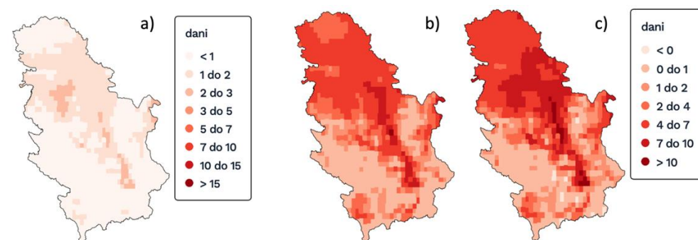
Слика Д1.2. Средњи број тропских дана по години ( TRD ) за референтни период 1961-1990 (лево), и промене TRD за периоде 2001-2020 (средње) и 2011-2020 (десно) у односу на вредности 1961-1990.
