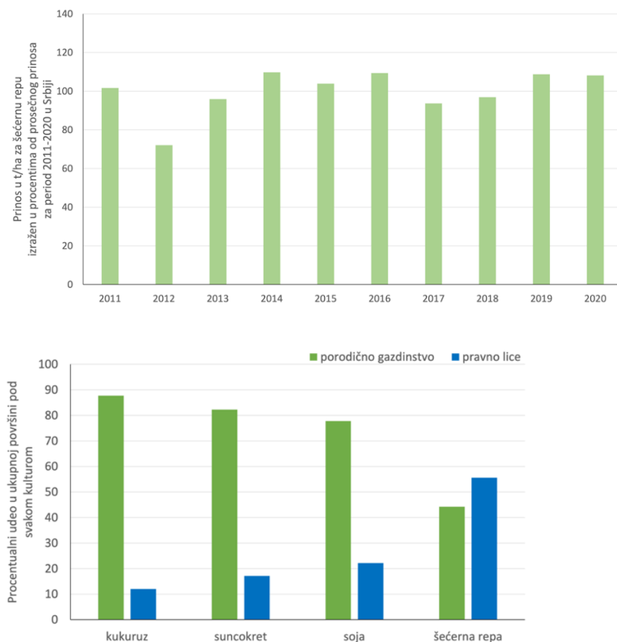
Слика Д2.24. Проценат од просечног приноса сунцокрета у т/ха у периоду 2011-2020 за сваку годину на територији Републике Србије (горњи панел). Удео површина под различитим културама по типу газдинства (доњи панел), за које су подаци ажурирани 2017. године.
